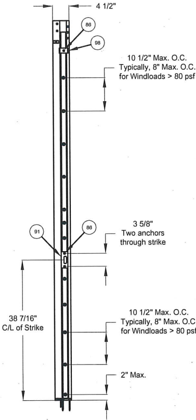
ACTIVE JAMB
