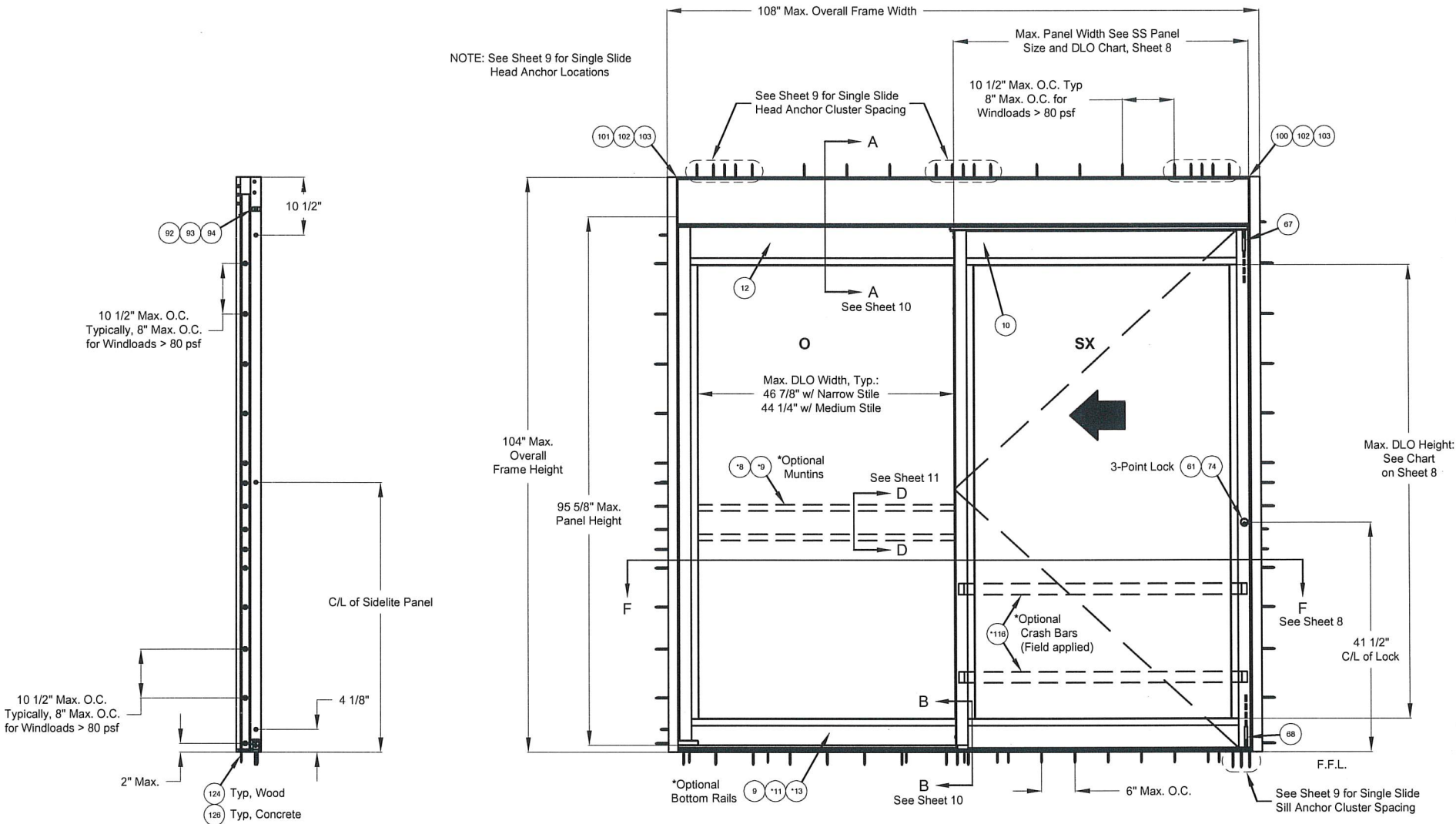
SIDELITE JAMB
